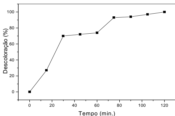
Figura 3. Descoloração (%) em função do tempo, obtida nas reações de fotocatalise utilizando-se o catalisador \text{TiO}_2 da Aldrich.
