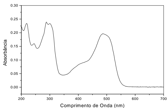
Figura 2. Espectro UV/Vis da solução aquosa 10 \text{ mg.L}^{-1} do corante reativo laranja-122.
